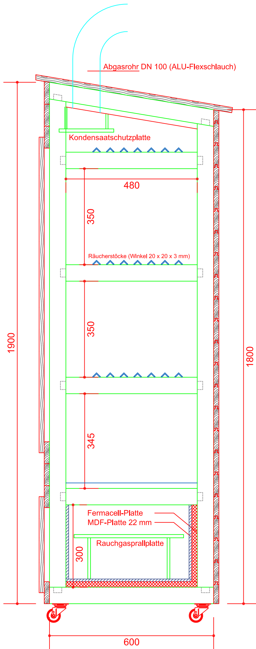
Seitenansicht
